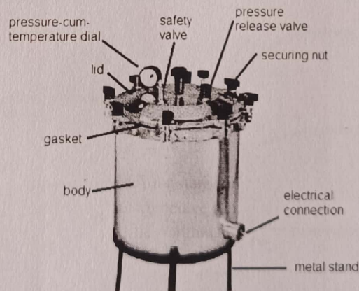
Fig. 1 Portable autoclave
