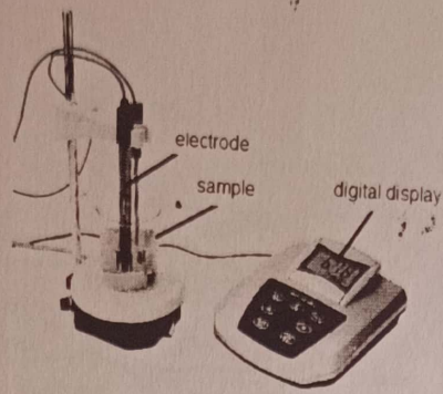
Fig 11 pH meter
