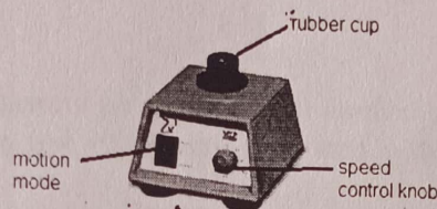
Fig. 5 Vortex mixer / shaker
