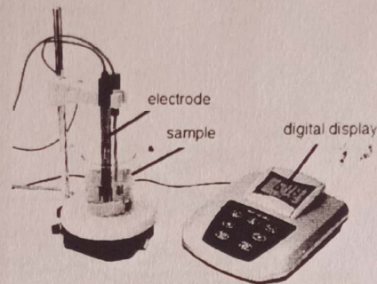
Fig. 11 pH meter
