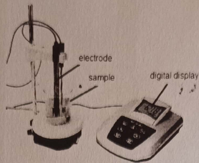
Fig. 11 pH meter
